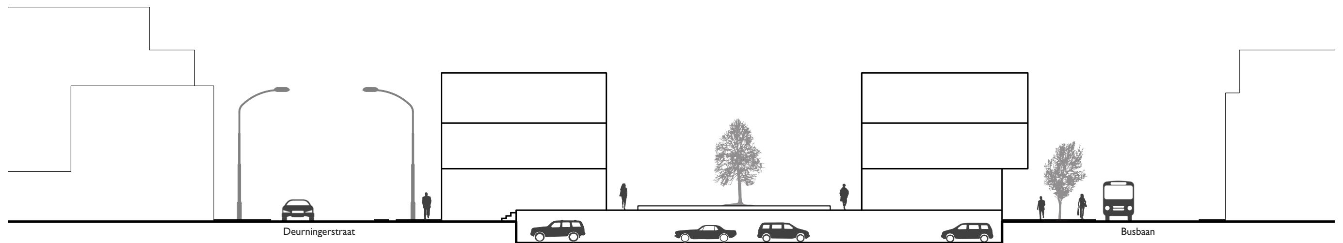
SCHEMATISCHE DOORSNEDE
